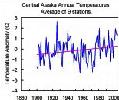
Nhiệt độ trung bình dựa theo dữ kiện gốc của NCDC [30]
