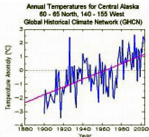
Nhiệt độ trung bình dựa theo dữ kiện điều chỉnh của GHCN [30]
